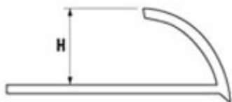
Ukončovací profil oblouček mosaz- odlehčený
